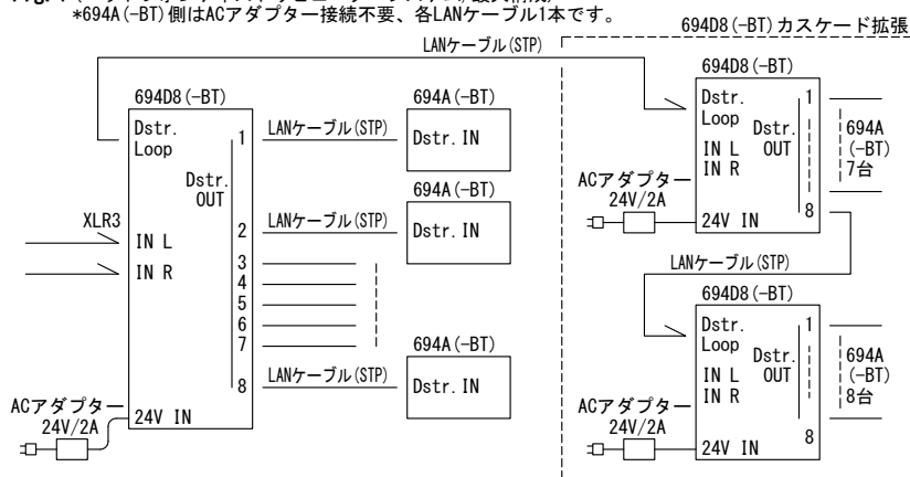
fig.1 (ヘッドフォンディストリビューターシステム/最大構成)
