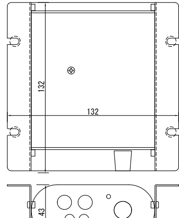
694A-BT 概観図
