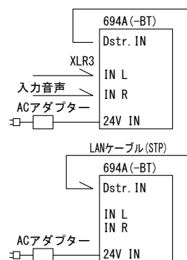
fig.2 (2台の場合はDstr. IN同士を接続します)
