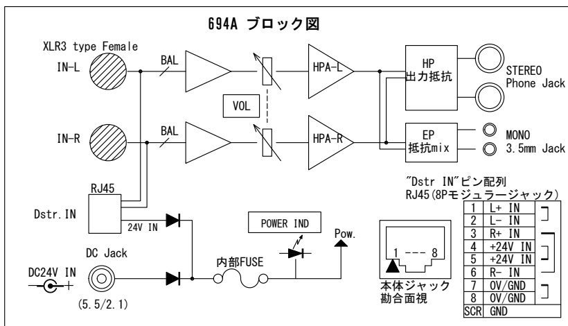
fig.2 (2台の場合はDstr. IN同士を接続します)
