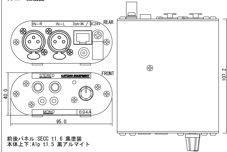
694A 概観図
