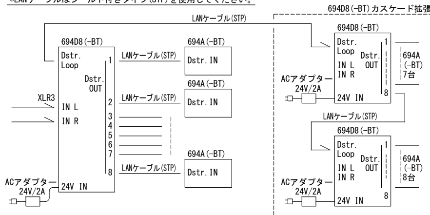
fig. 1 (ヘッドフォンディストリビューターシステム/最大構成)
